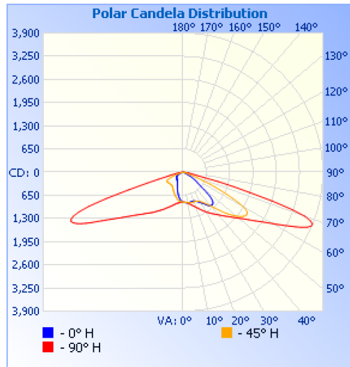
NEPTUNE-40W-30K-T2
